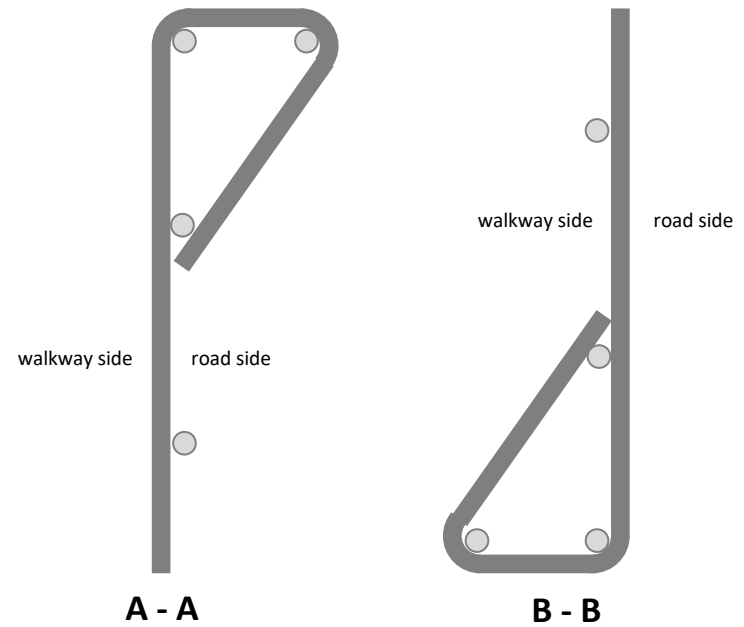
REKABENTUK DAN BUTIRAN 'GALVANIZED FENCING'
